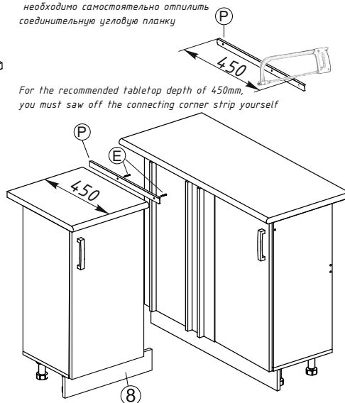
Цоколь обрезан в нужный размер Socle of the right size
