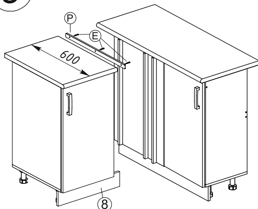
Цоколь обрезан в нужный размер Socle of the right size
