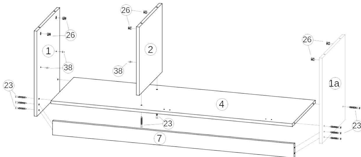
Рис.1 Сборка тумбы
