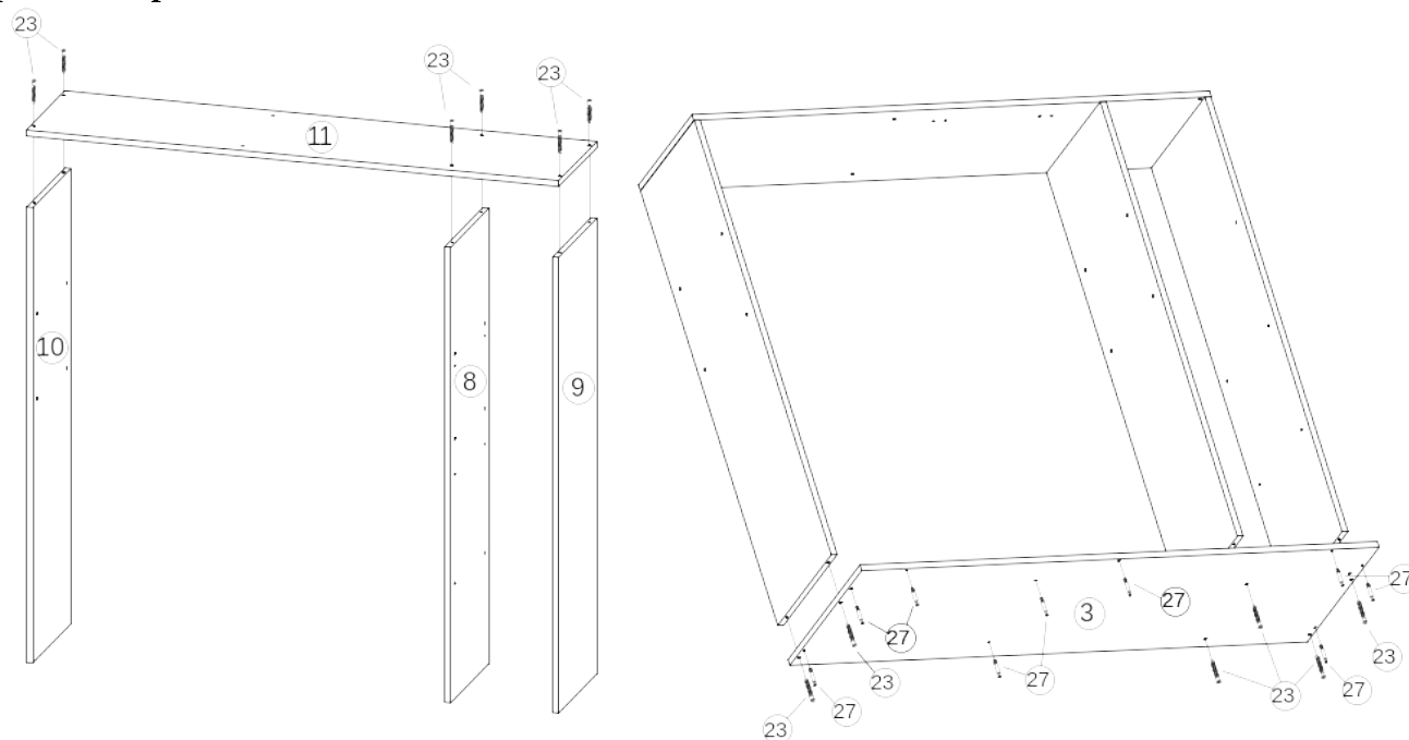
Рис.2 Сборка надстройки
