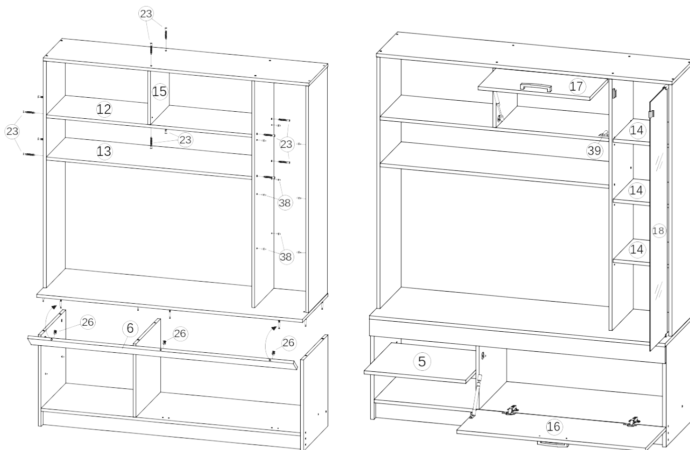
Рис.3 Окончательная сборка
