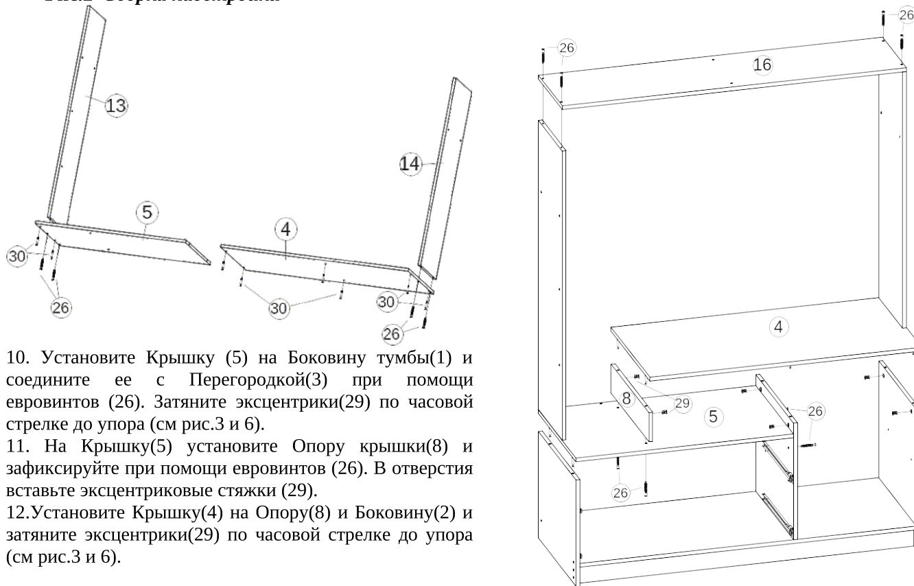
Рис.2 Сборка надстройки
