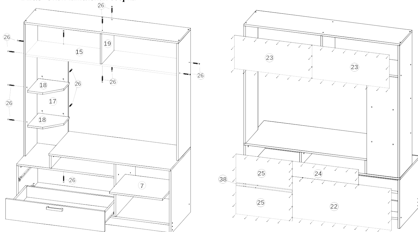
Рис.3 Окончательная сборка
