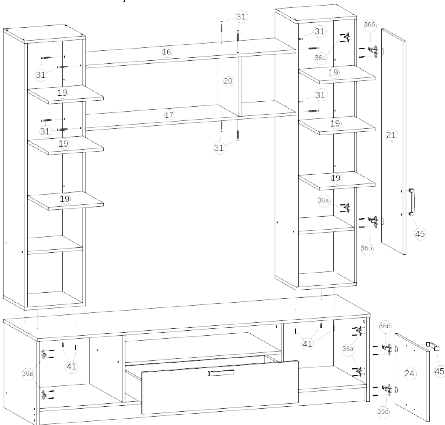
Рис.3 Окончательная сборка
