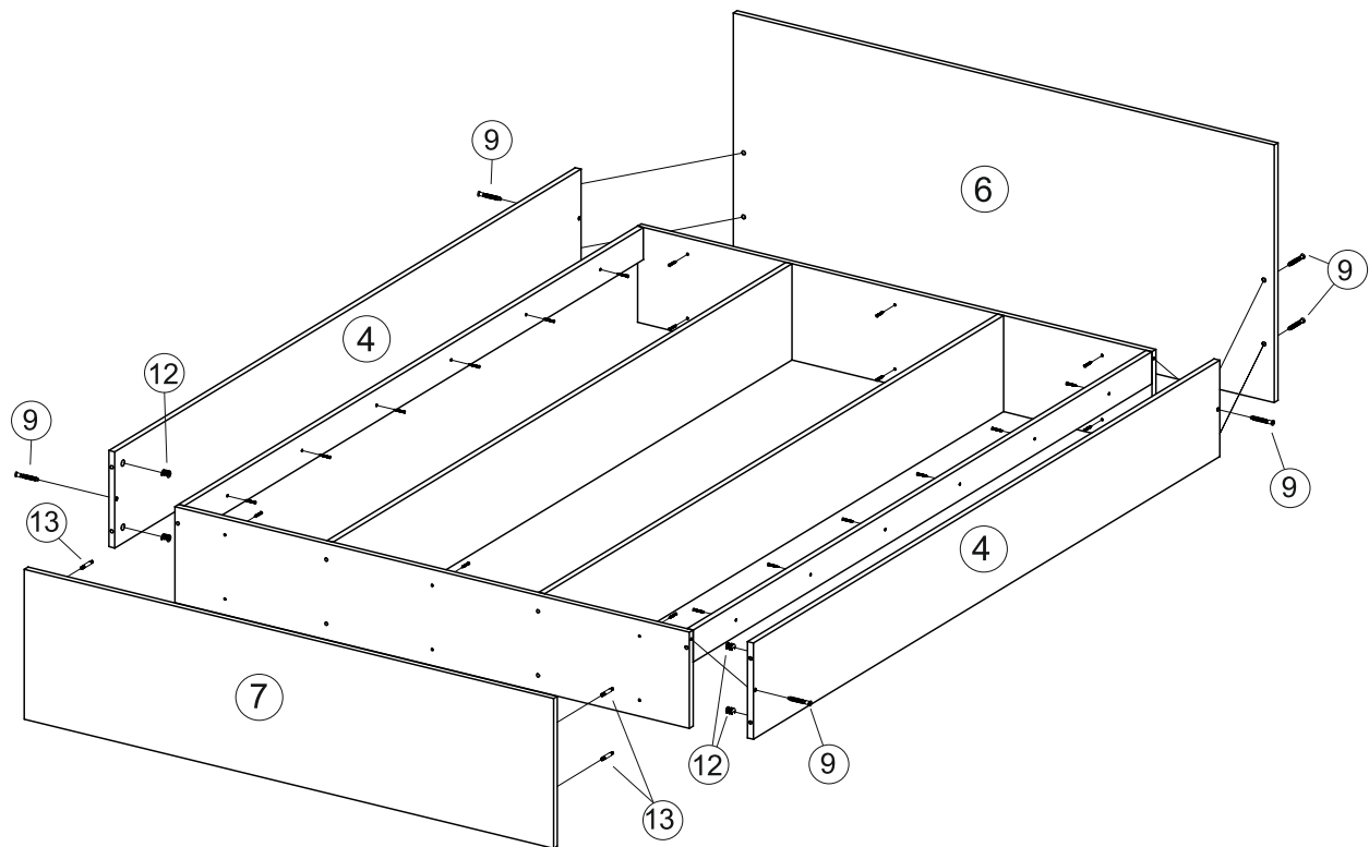
Рис.4 Окончательная сборка
