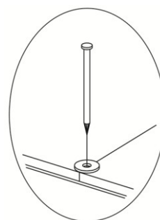
Рис.3 - Монтаж задних стенок на стыке На рисунке показаны Гвоздь+Шайба
