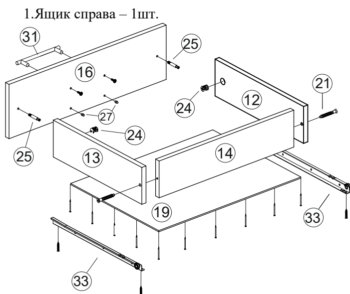
Рис.5 Сборка ящиков
