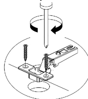
Рис.9 - Монтаж чашки петли 28а на фасад
