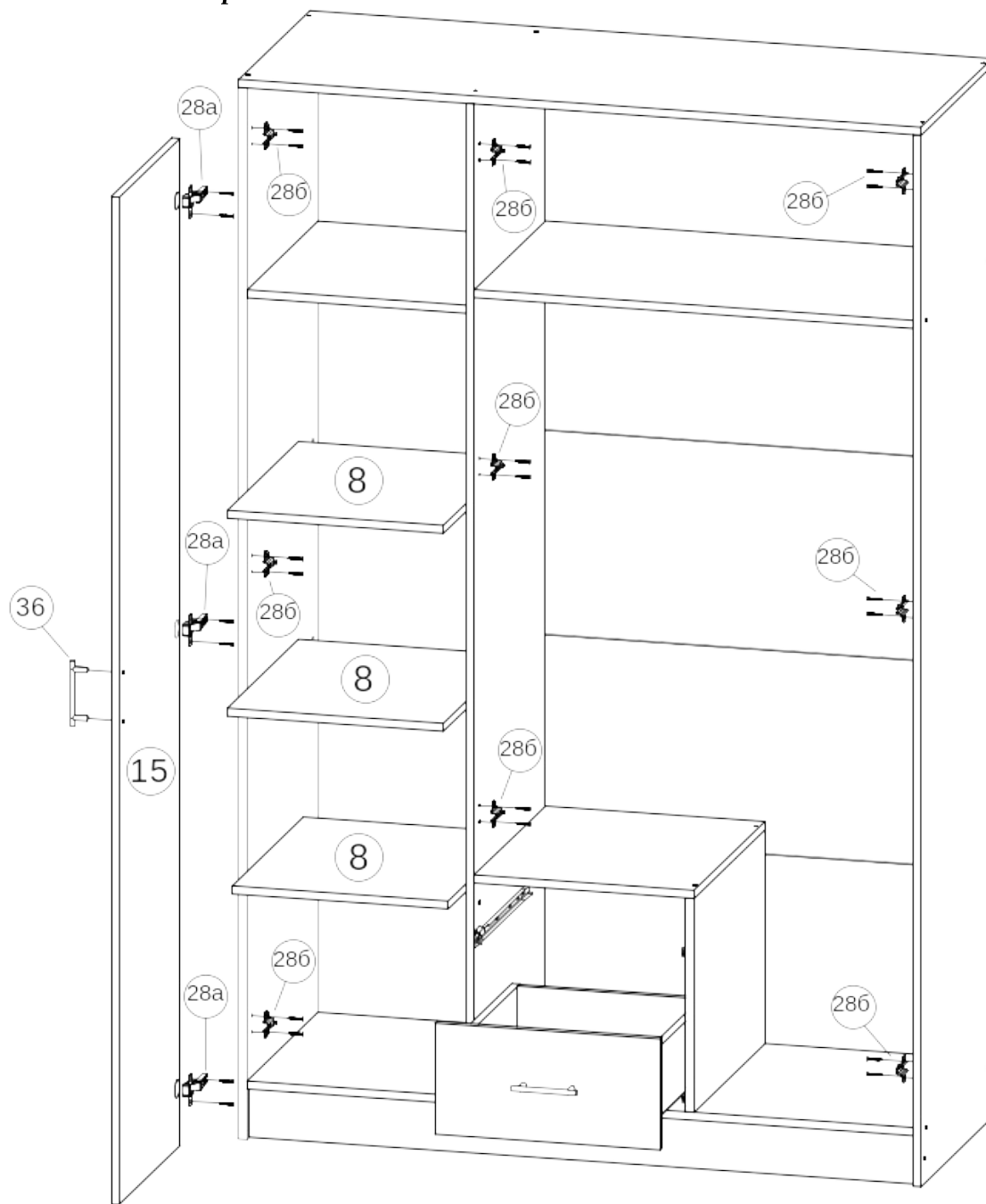
Рис.8 - Монтаж крестовины петли 28б на боковину
