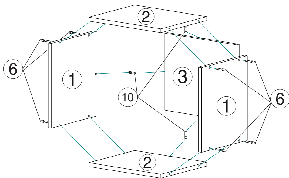
Рис.1 Сборка полки ПЛВ 400
