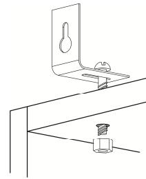
Рис.5 Монтаж навеса
