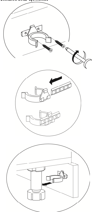
Рис.16 Монтаж клипс и установка цоколя
