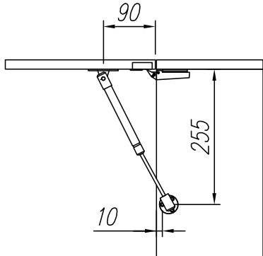
Рис.6 Монтаж крепежных планок газлифта
