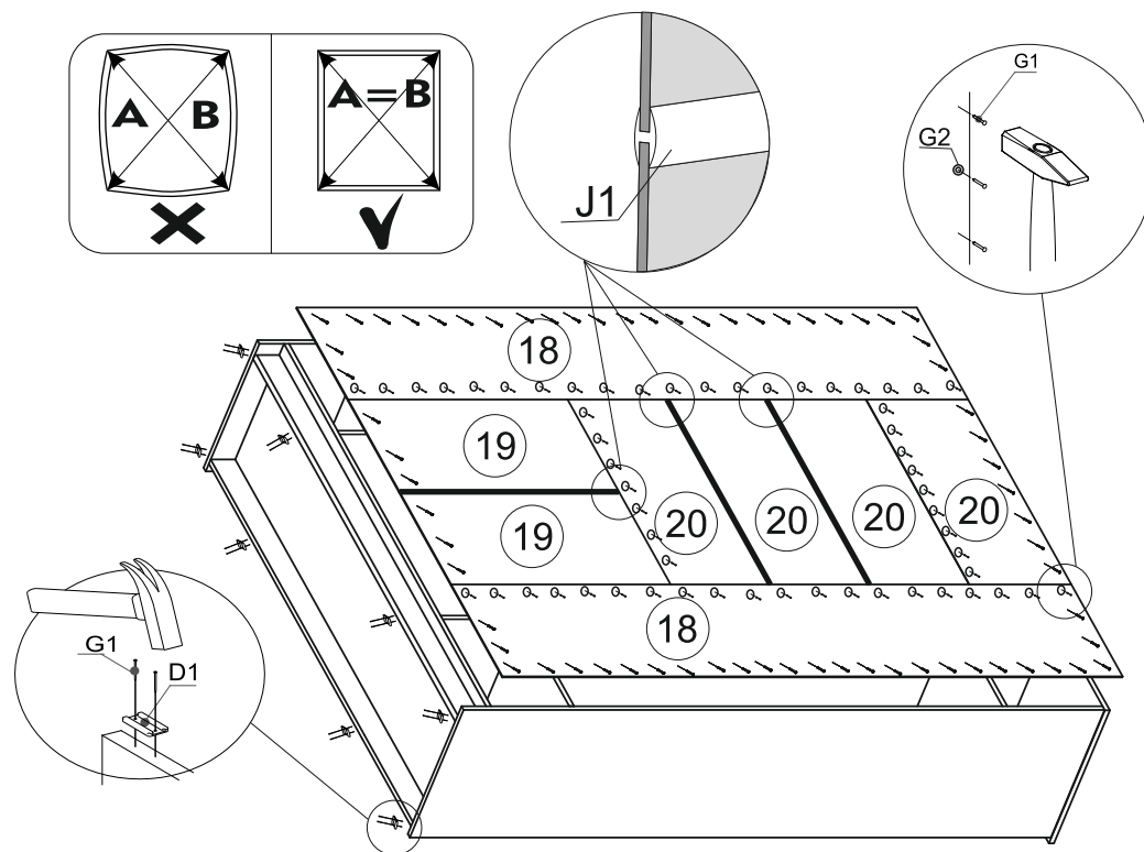
Схема монтажа навеса Installation diagram of the canopy
