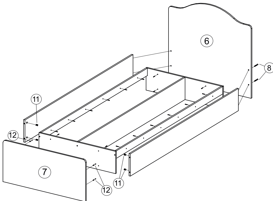
Рис.3 Окончательная сборка
