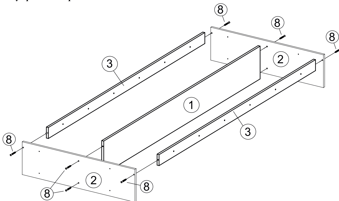
Рис.1 Сборка внутреннего каркаса
