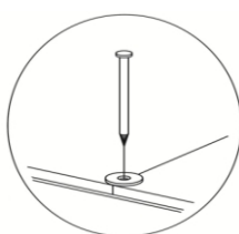
Рис.5 - Монтаж задних стенок на стыке На рисунке показаны Гвоздь+Шайба
