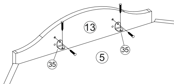
Рис.9 - Монтаж Карниза на крышу
