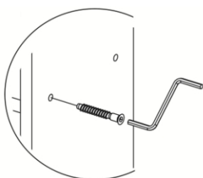
Рис.4 - Установка евровинта
