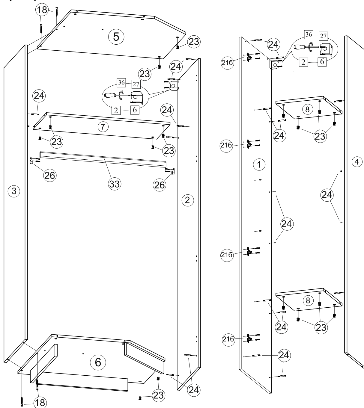
Рис.2 Сборка каркаса
