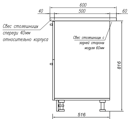
Схема монтажа столешницы
