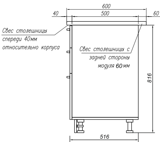
Схема монтажа столешницы
