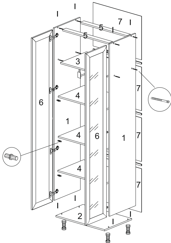
Комплектующие детали секции №3
