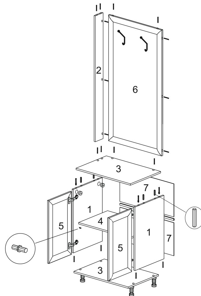
Комплекующие детали секции 2
