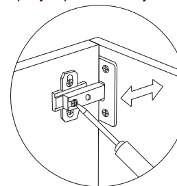
регулировка по глубине
