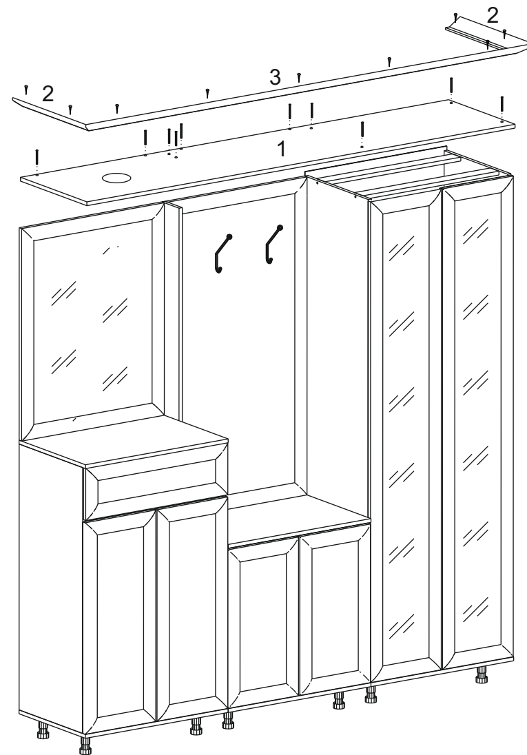
Комплектующие детали при установке крышки
