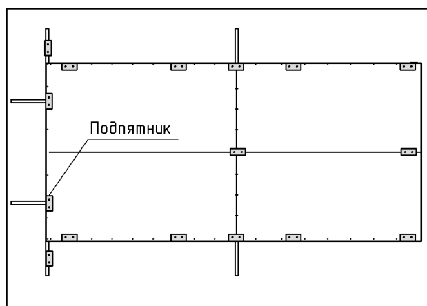
Схема 2. Крепление подпятников к корпусу кровати
